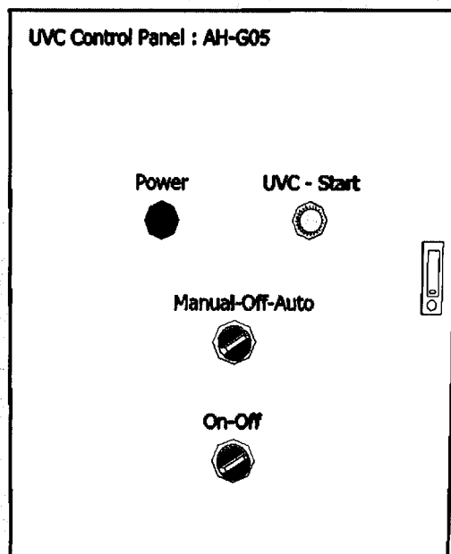
รูปภาพตัวอย่างหน้าตู้ : ควบคุมระบบฆ่าเชื้อระบบหลอดไฟแสง UV-C ประจำเครื่องส่งลมเย็น
